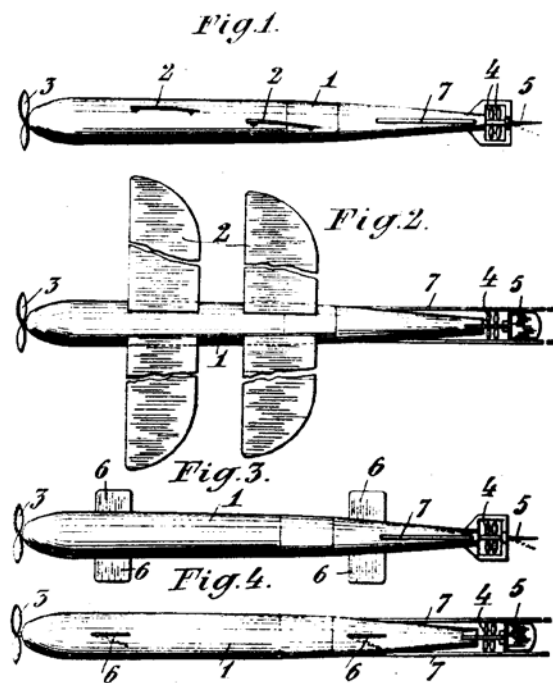
Plany techniczne J. Warchałowskiego
