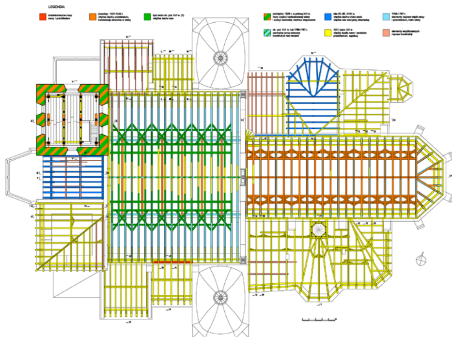
Więźba dachowa nad prezbiterium
